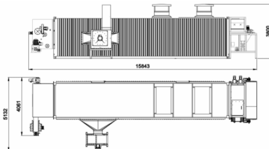
Rysunek 1 Automatyczna taśmowa suszarnia produktów sypkich typu ATSS-1/400
